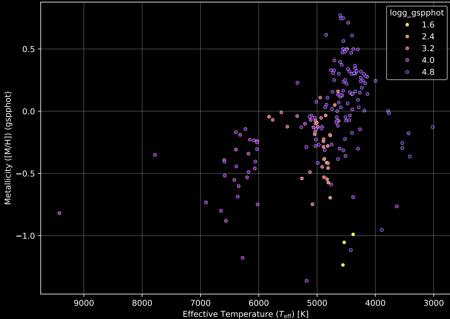
APOGEE DR17 Field: [150+60] Stellar Population Parameters (n= 185)
